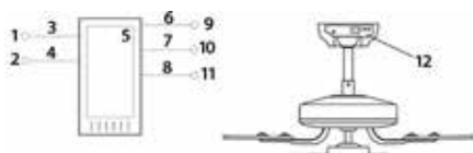
Diagramma collegamenti ricevitore
